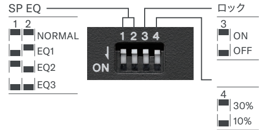
セットアップスイッチでEQ設定・マスキング設定が可能
